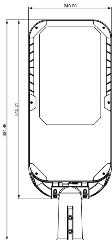
主视图
